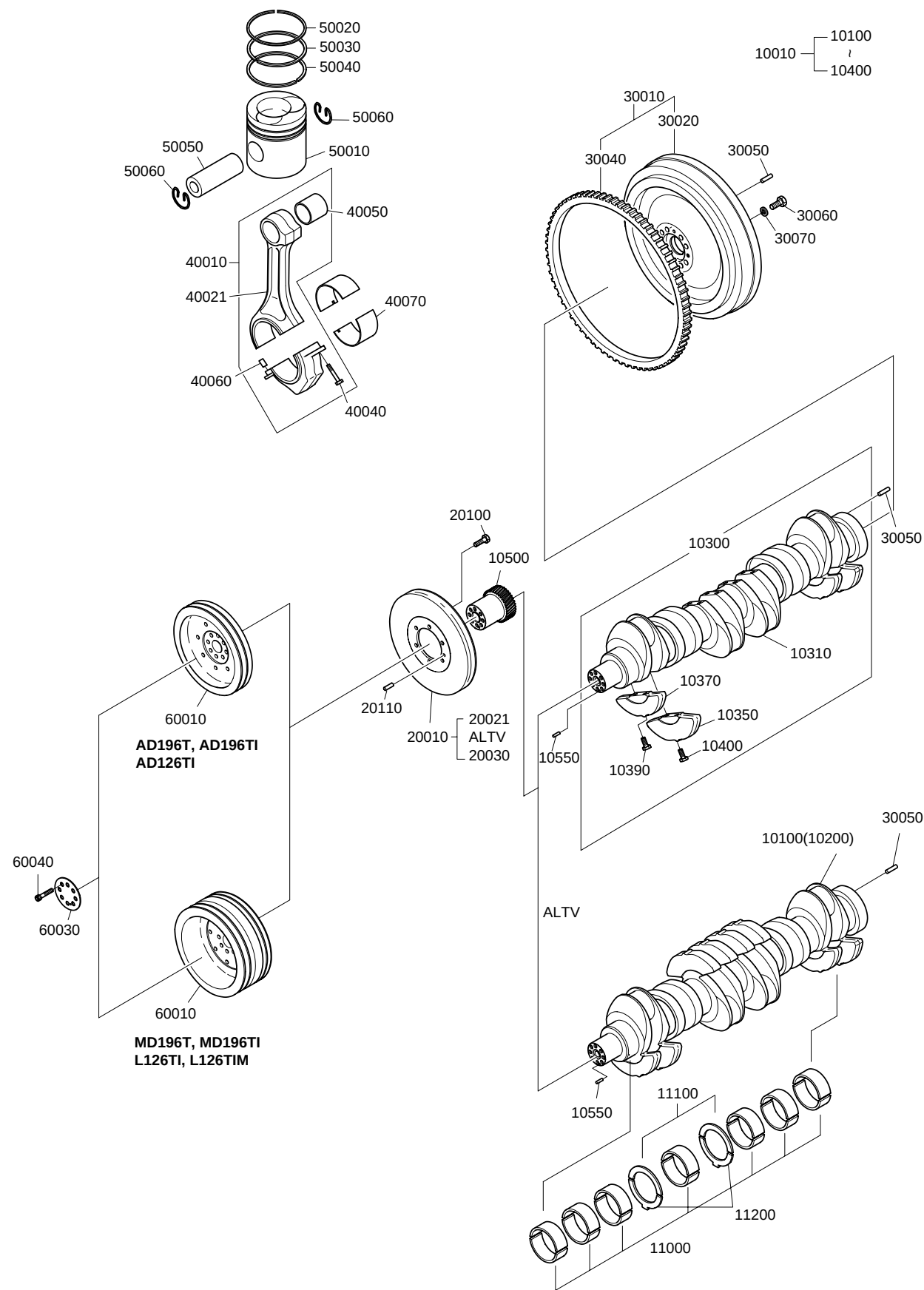
구동 장치 Fig.003 DRIVING SYSTEM
